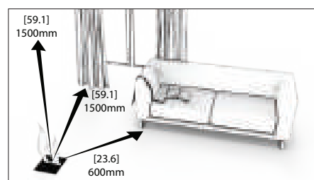
Dégagements Intérieur
